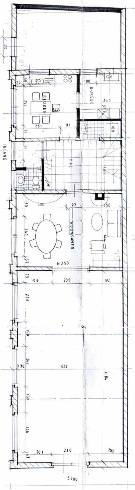
GRONDPLAN
